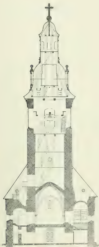
Fig. 20. Tvärsektion genom tornpartiet. Efter uppmätning av S. Curman o. A. Roland 1907, kompletterad av H. Sundberg 1927.
